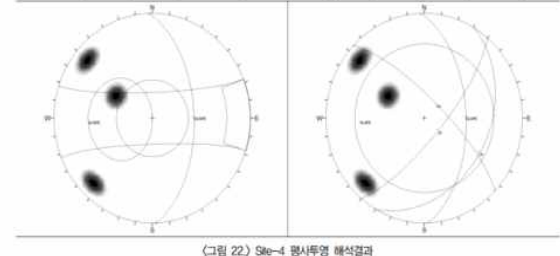
〈그림 22〉 Site-4 평사투영 해석결과
